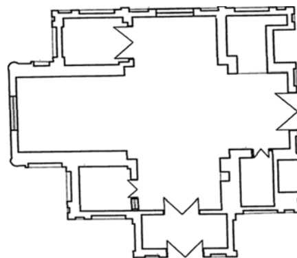
شکل ۳: پلان امامزاده سراج‌الدین (آرشیو میراث فرهنگی استان آذربایجان غربی)
