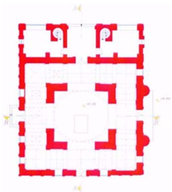
شکل ۱: پلان امام‌زاده محمد و ابراهیم ارومیه (مأخذ، آرشیو سازمان میراث فرهنگی استان آذربایجان غربی)
