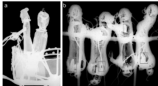
تصویر ۴- جزئیاتی از رادیوگرافی ایکس تصویر ۳ را نشان می‌دهد، مغزهای میان‌تهی از: (a) پیکره‌ها در ارايه و (b) اسبها.
